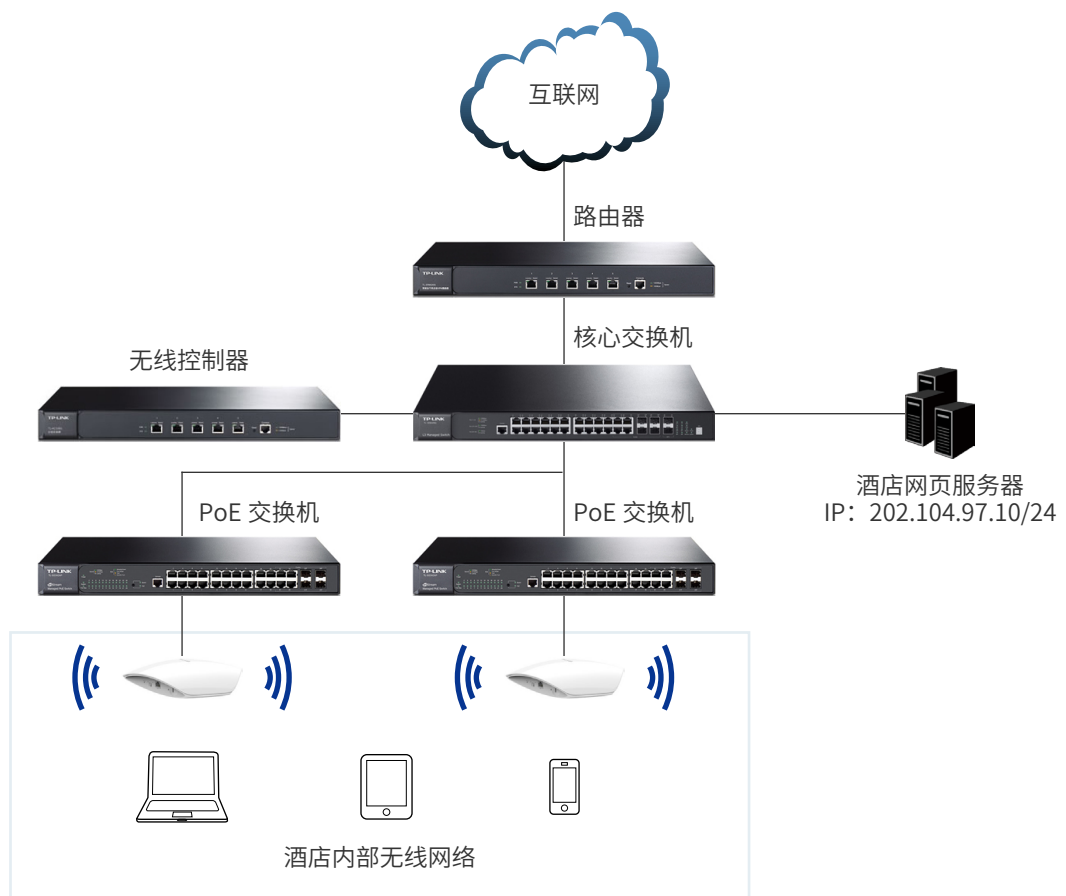
图 6-43 酒店无线网络应用拓扑
