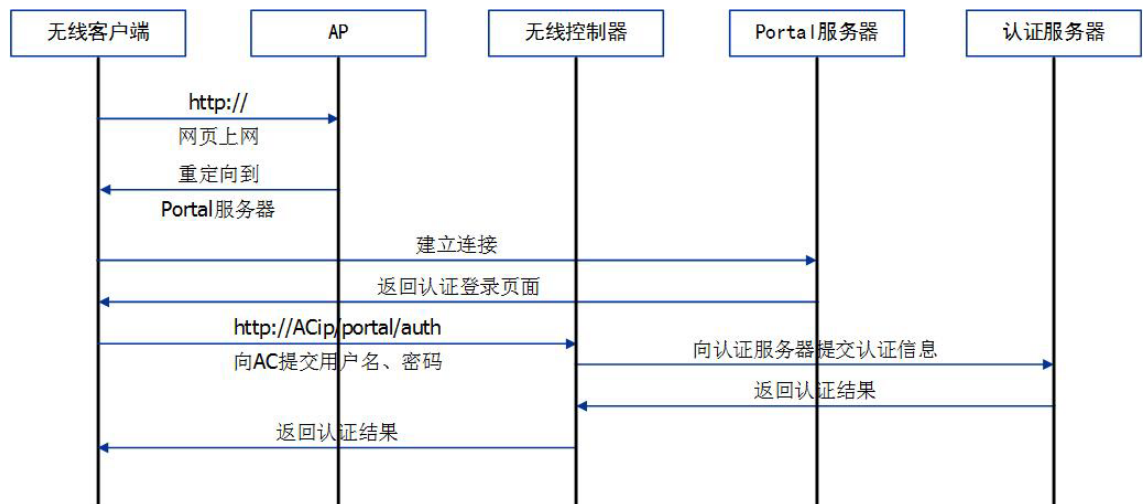
图 6-12 Web 认证过程示意图
