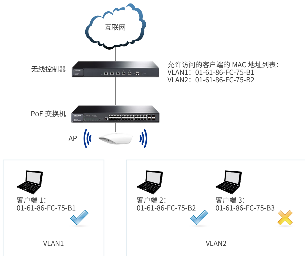
图 6-1 MAC 认证拓扑图
