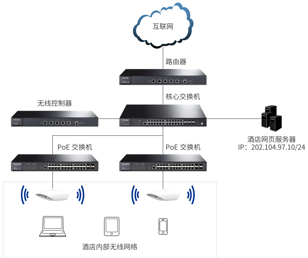
图 6-38 酒店无线网络应用拓扑
