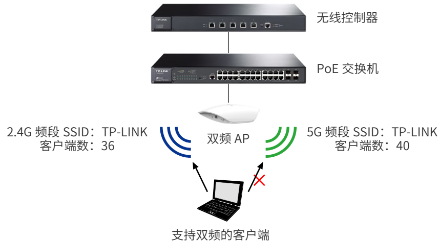
图 4-4 频谱导航应用场景
