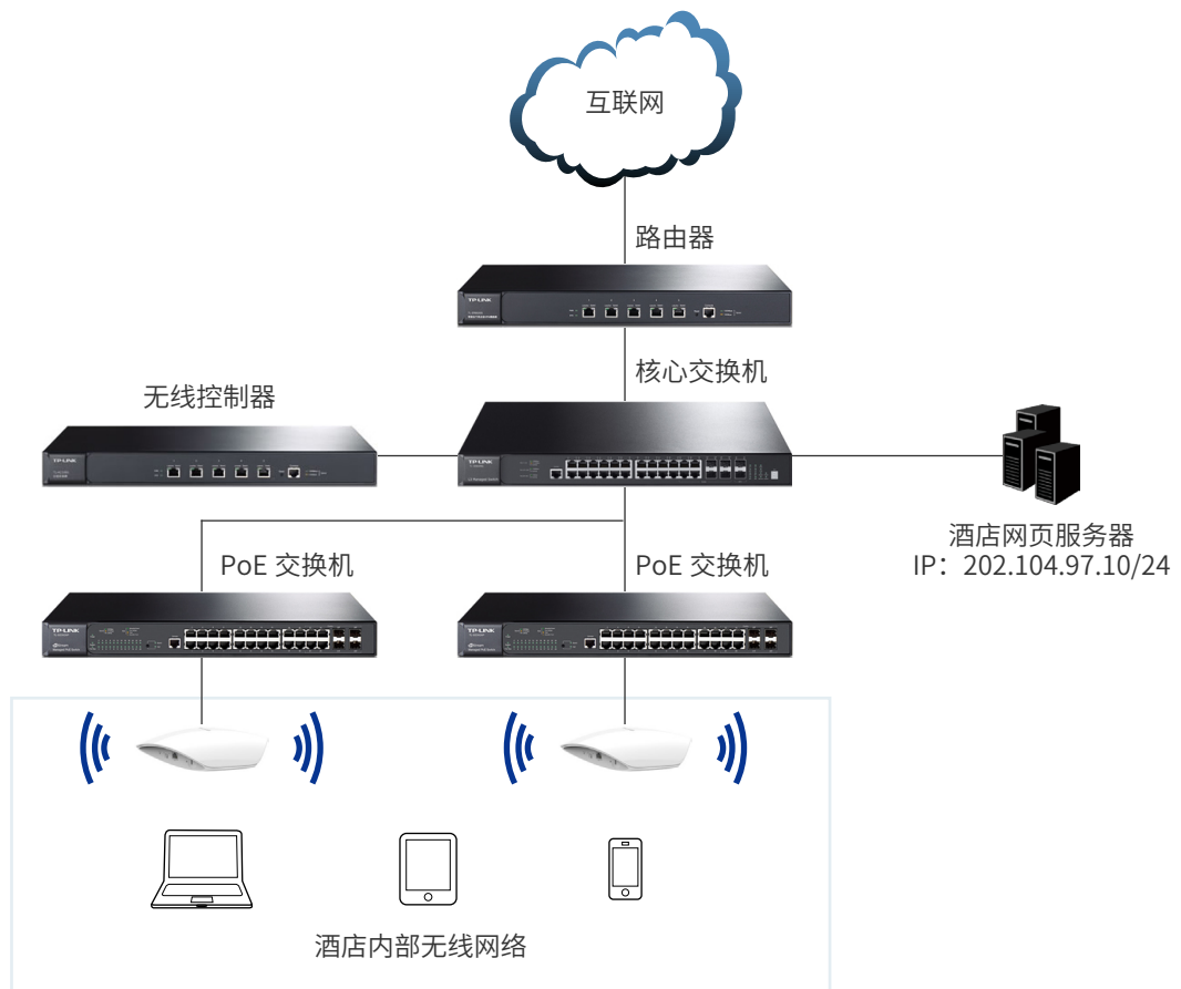
图 6-34 酒店无线网络应用拓扑
